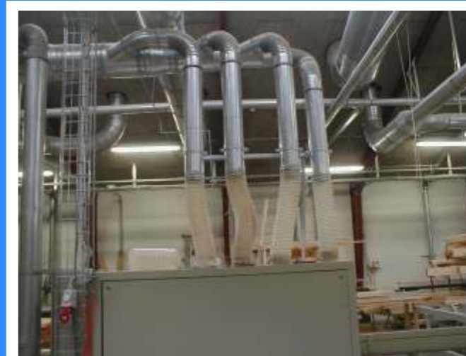
Eksempel på tilslutning af spåtagningsmaskine
